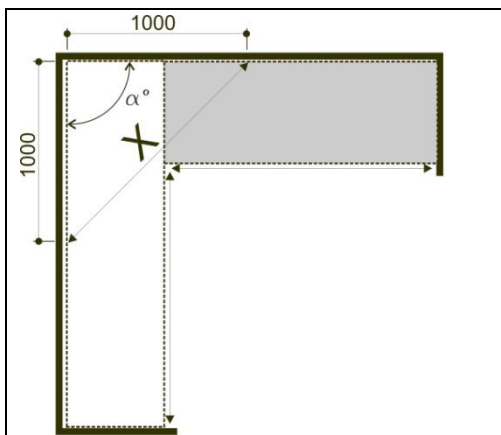
Рис.1. Угол 90^\circ X = 1414 мм
