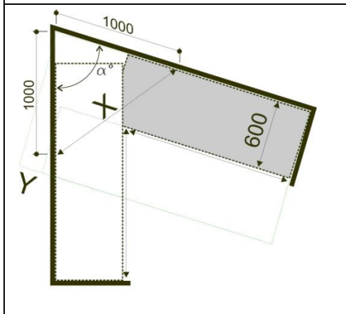
Рис3. Если X меньше 1414 мм, то угол острый, меньше 90^\circ . Длина помещения, измеренная по стене, будет больше длины, измеренной на расстоянии 600 мм от стены на Y .
