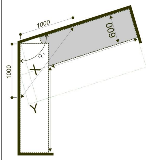
Рис.2. Если X больше 1414 мм, то угол не является прямым, он больше 90^\circ . Длина помещения, измеренная по стене, будет меньше длины, измеренной на расстоянии 600 мм от стены на Y .
