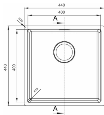
ОНМ 400 мойка ОПТИМА-НМ в стол от 500 мм. Внешние размеры 440х440х205
