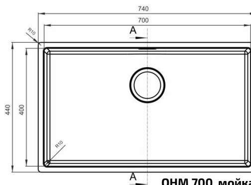
ОНМ 700 мойка ОПТИМА-НМ в стол от 800 мм. Внешние размеры 740х440х205
