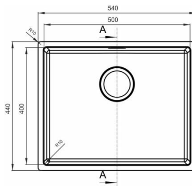
ОНМ 500 мойка ОПТИМА-НМ в стол от 600 мм. Внешние размеры 540х440х205
