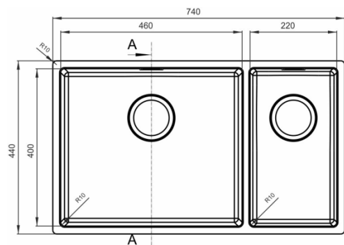
ОНМ 460/220 мойка ОПТИМА-НМ в стол от 800 мм. Внешние размеры 740х440х205
