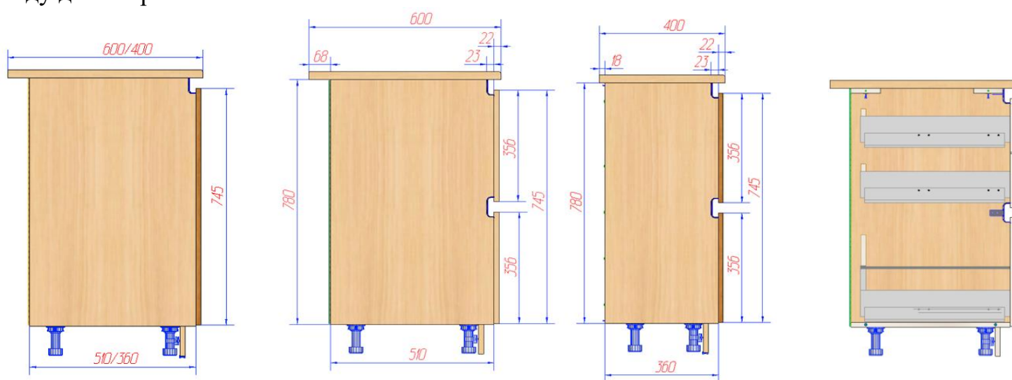
Рис.1 Габариты столов
